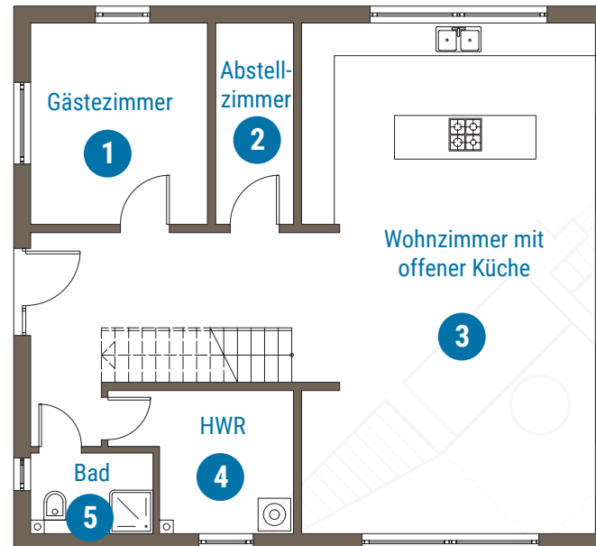
ERDGESCHOSS 5 RÄUME
