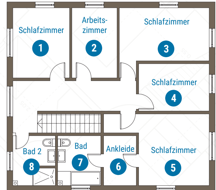
1. OBERGESCHOSS 8 RÄUME
